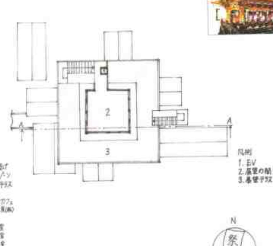
3階平面図 Scale 1:300
