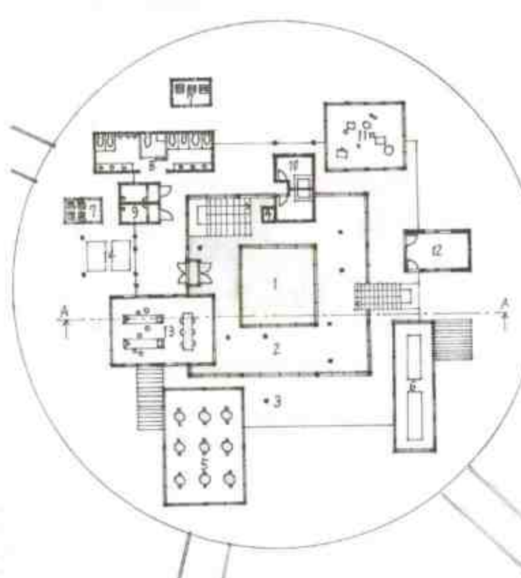
配置図兼1階平面図 Scale 1:300
