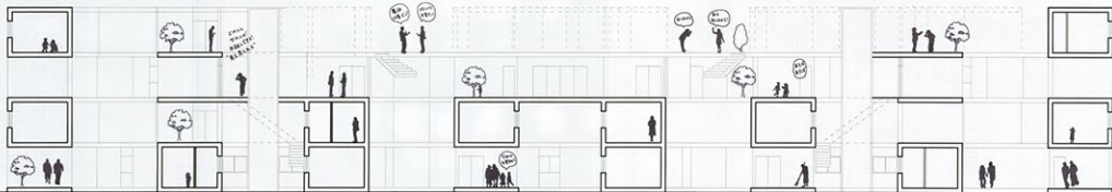
A-A断面図 S=1/100
