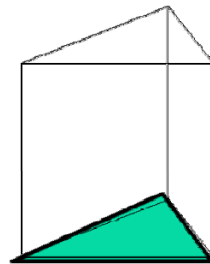
int
