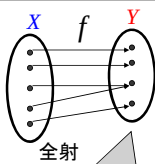
全射
