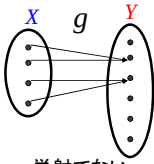
単射でない
