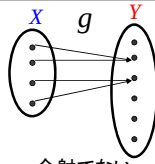
全射でない
