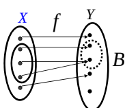
f^{-1}(B)
