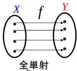
全単射
