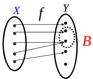
f^{-1}(B)
