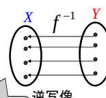
逆写像
