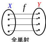
全単射
