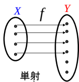
単射
