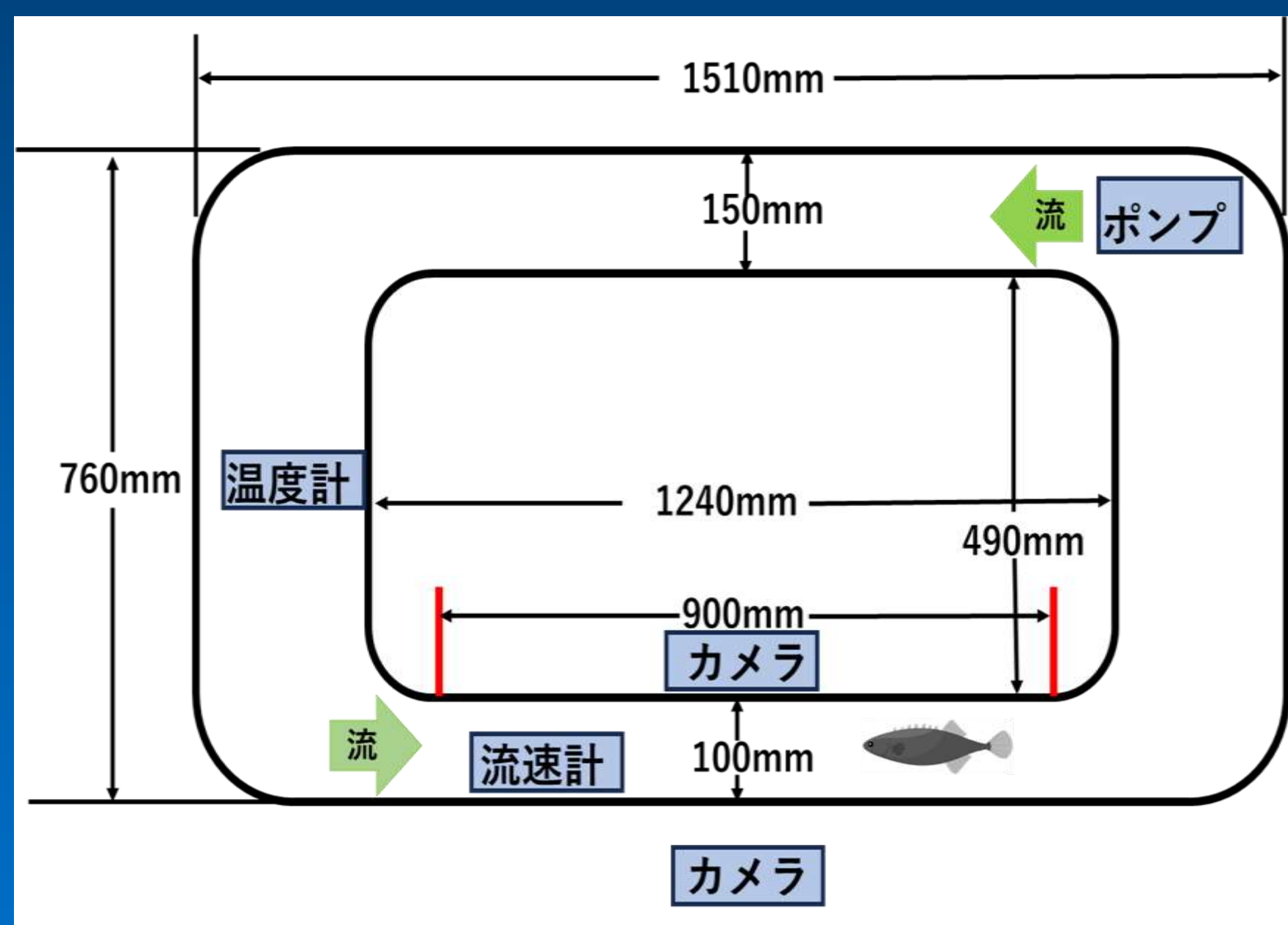
図-1 回流型開水路
